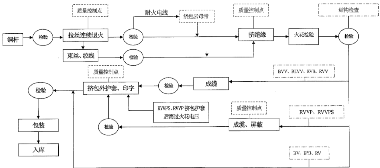
图3-1 生产工艺流程图
